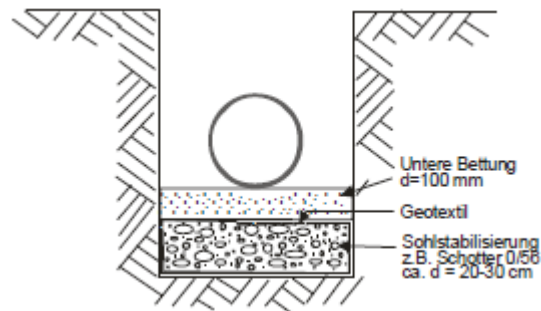
Bild 4: Sohlstabilisierung mit Schotter
