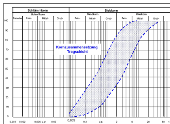
Bild 5: Bandbreite des zu verwendenden Korngemisches
