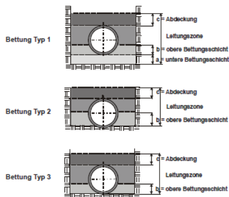
Bild 3: Ausführung der Bettung nach DIN EN 1610
