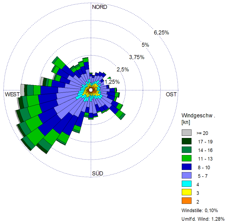
Abb. 3 Darstellung der Windrichtungsverteilung und Windgeschwindigkeiten, gemessen an der Wetterstation Bremervörde (akt 2004)
